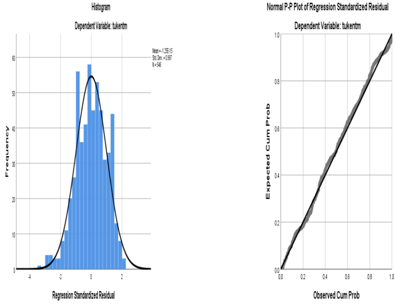
Şekil 2: Standart regresyon yükü frekansları
